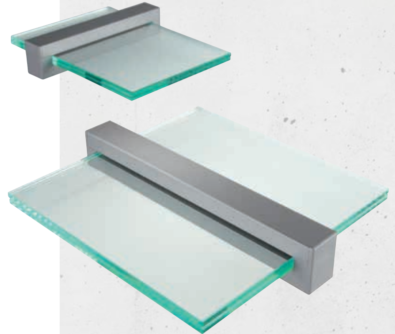
A 1 oder 2 Glasplatten B optional Beschriftungseinlage C Adapter-Basis D Basis-Abdeckung E Glashalter F Frontabdeckung
