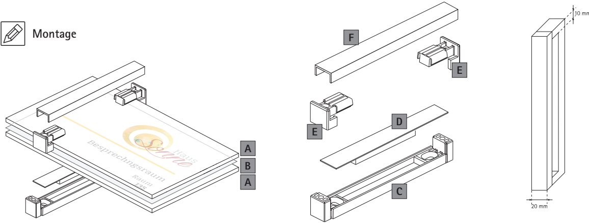
A 1 oder 2 Glasplatten B optional Beschriftungseinlage C Adapter-Basis D Basis-Abdeckung E Glashalter F Frontabdeckung
